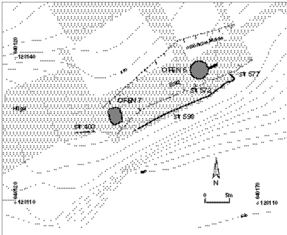
25: Schematischer Plan der Öfen bei der «Waldmatte». Die Öfen sind in der Einfüllung einer Spalte karstischen Ursprungs eingetieft. Gestrichelte Linie: Verlauf der Mulde; bell gerastert: ausgegrabene Flächen. Plan schématique des fours du secteur de «Waldmatte». En trame claire: surfaces fouillées. Les «L» représentent la faille d'origine karstique comblée, dans laquelle les fours ont été implantés.
